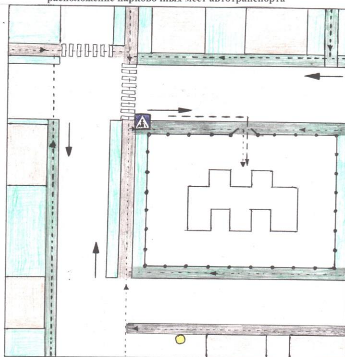
1.2. Схема организации дорожного движения в непосредственной близости от образовательного учреждения с размещением соответствующих технических средств, маршруты движения детей и расположение парковочных мест автотранспорта
